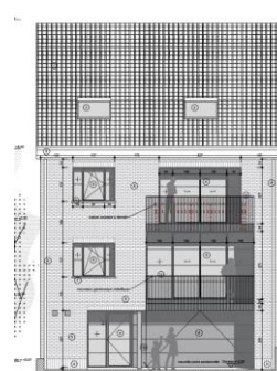
Élévation projetée. Image tirée du dossier.
